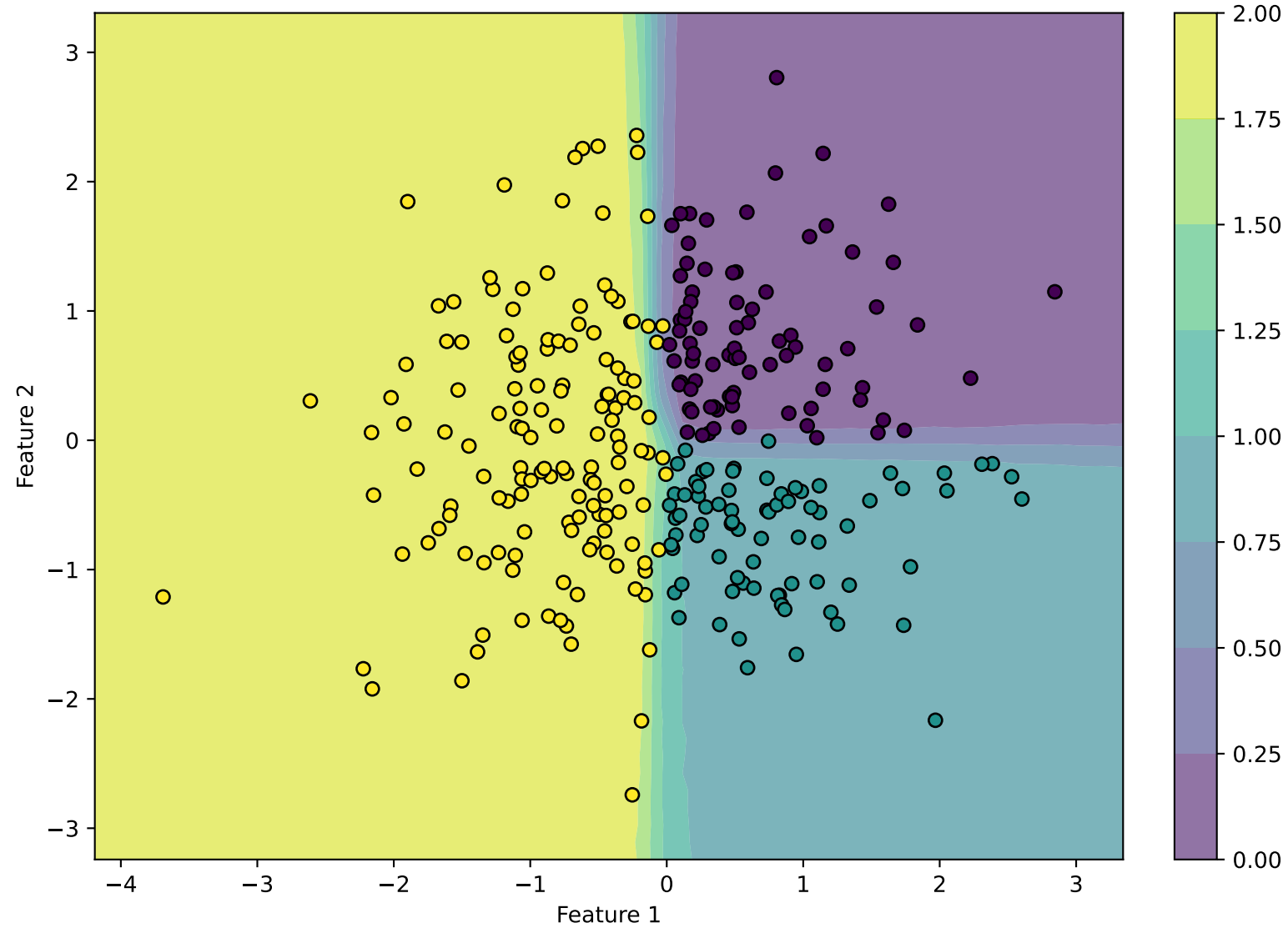
Posterior Predictive Mean
